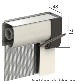
Système de blocage du coffre avec clé allen
